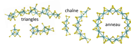
Différents types de nano-agrégats représentatifs de la phase amorphe MoS 3 .
