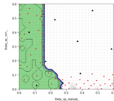
Pour deux paramètres de contrôle, estimation (en vert) du domaine de respect de la norme d'émissions de NH 3 (points initiaux simulés en noir, points ajoutés par la méthode itérative en rouge).
